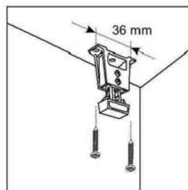
Mennyezeti szerelés
