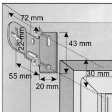
Homlokfalas szerelés
