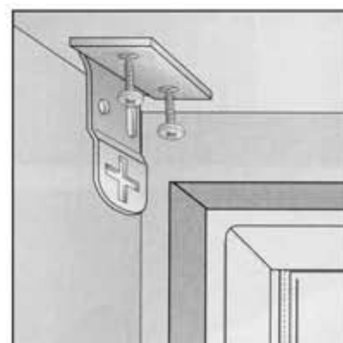
Mennyezeti szerelés
