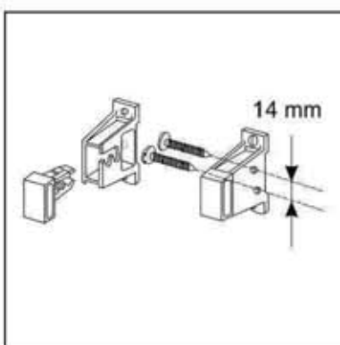
Oldalfalas szerelés
