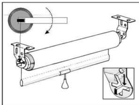
Mennyezeti szerelés
