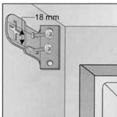
Oldalfalas szerelés
