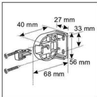
Homlokfalas szerelés
