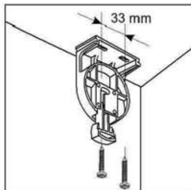
Mennyezeti szerelés
