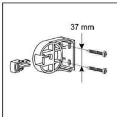
Oldalfalas szerelés
